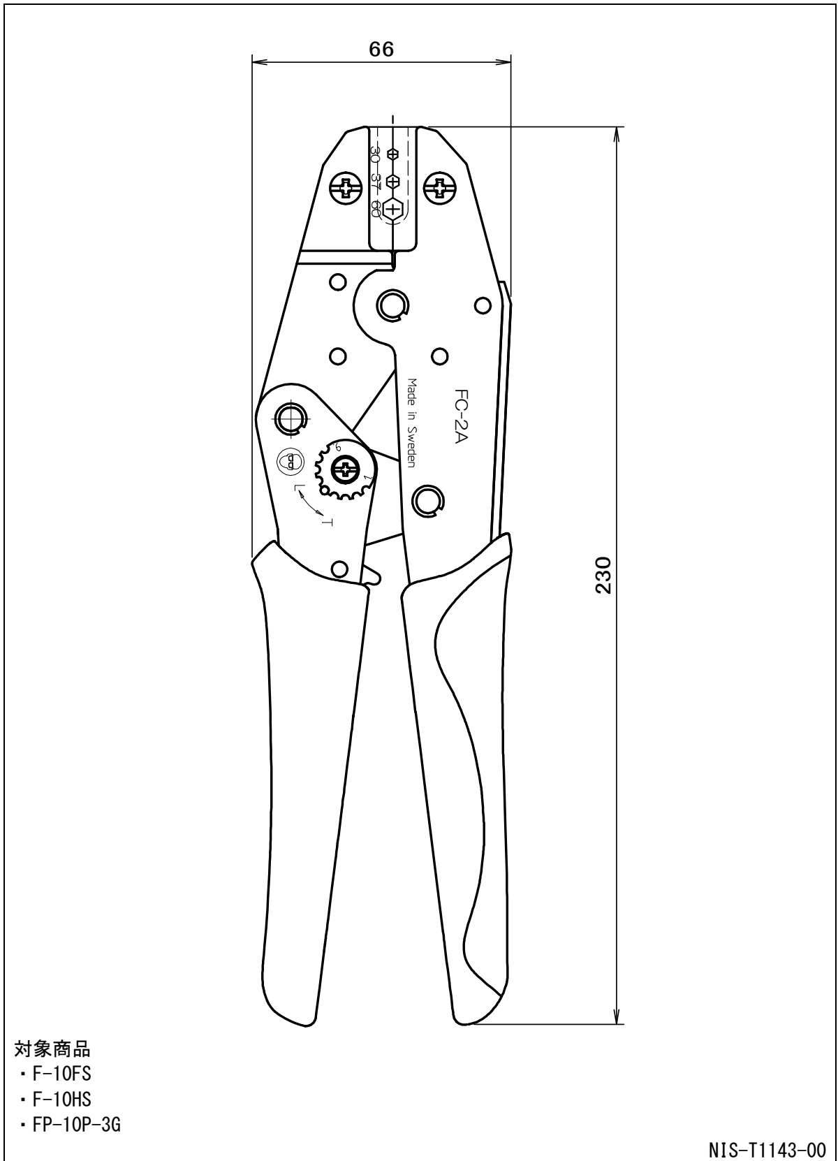
外觀圖 FC-2A
