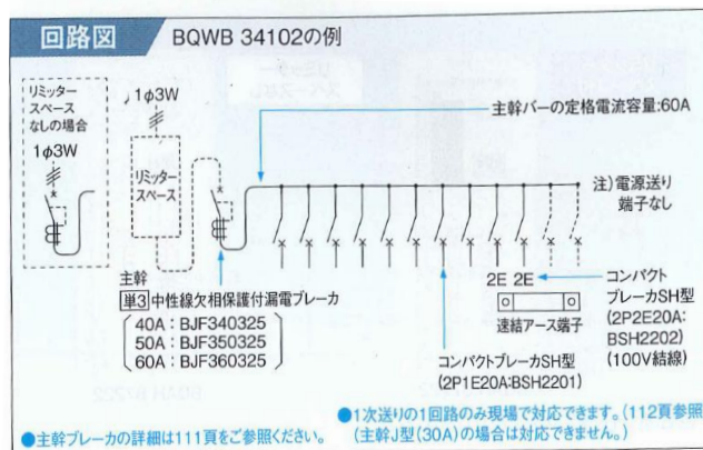
【図2】BQWB 34102 回路図
